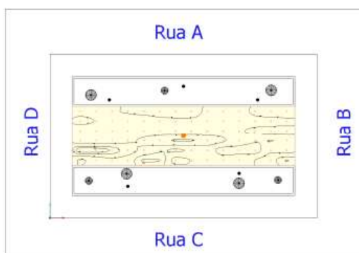
Figura C.5 – Imagem da praça com destaque para a superfície de cálculo com os (14 x 6) pontos e as linhas de iso-iluminância
