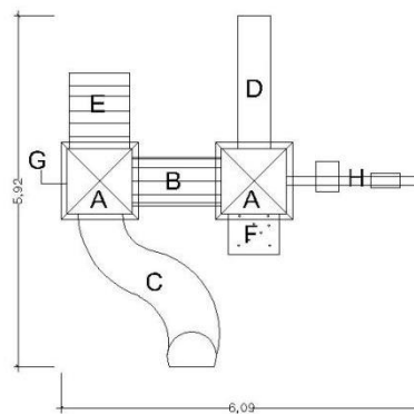
PLAYGROUND - 02 TORRES COBERTAS MODELO 02
